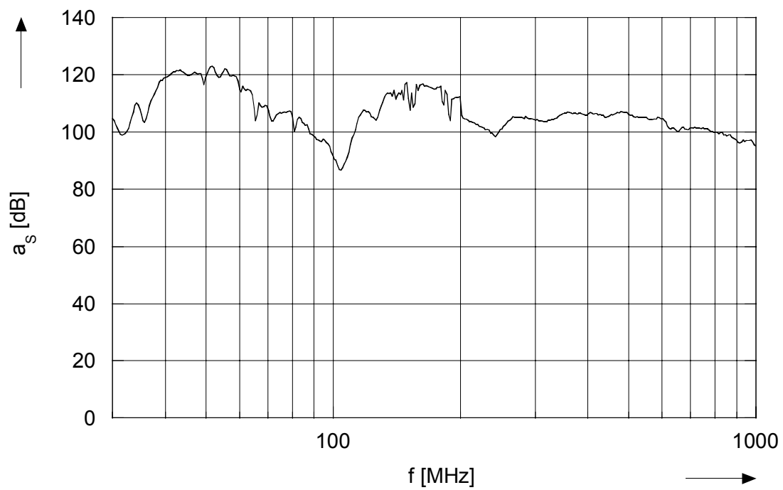
Bild 3: Messdynamik für die Schirmdämpfungsmessungen im Frequenzbereich von 30 MHz bis 1 GHz (vertikale Polarisation der Sendeantenne).
