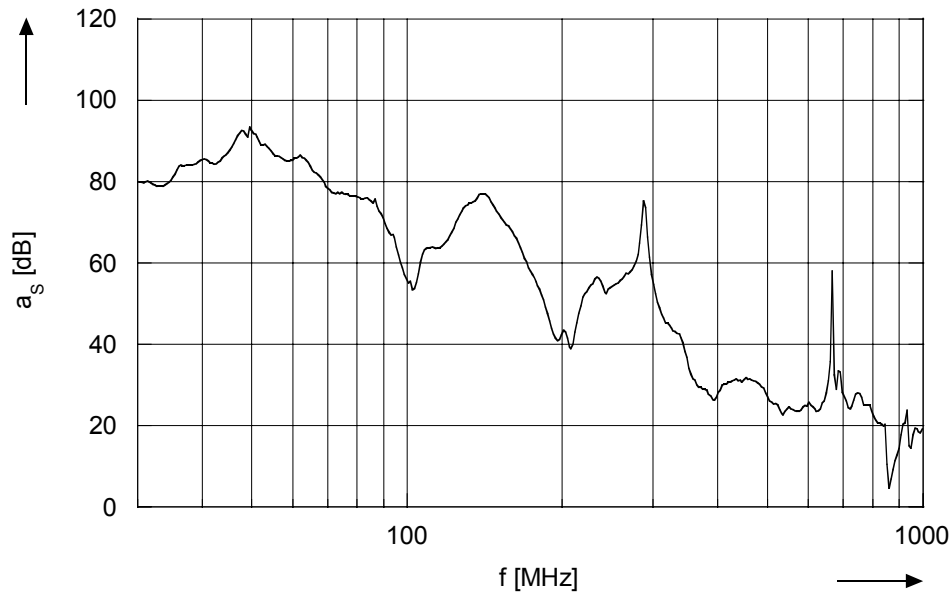
Bild 9: Schirmdämpfung im Bereich von 30 MHz bis 1 GHz, „Ratiopac pro ungeschirmt“, Einstrahlung auf die Frontseite, Polarisation vertikal.
