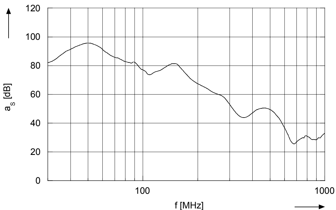
Bild 8: Typische Schirmdämpfung im Bereich von 30 MHz bis 1 GHz, „Ratiopac pro geschirmt“. Berechnet aus Worst Case der Kurven der Seitenwände, wobei Hohlraumresonanzen durch Glättung ausgeblendet wurden.
