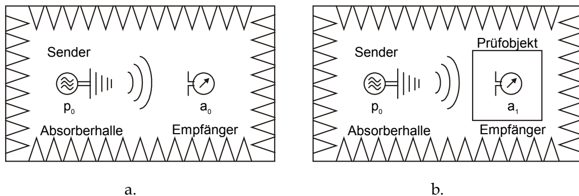
Bild 2: Messung der Einfügungsdämpfung technischer Schirmhüllen (Prinzip). a) Messung ohne Prüfobjekt, b) Messung mit Prüfobjekt.
