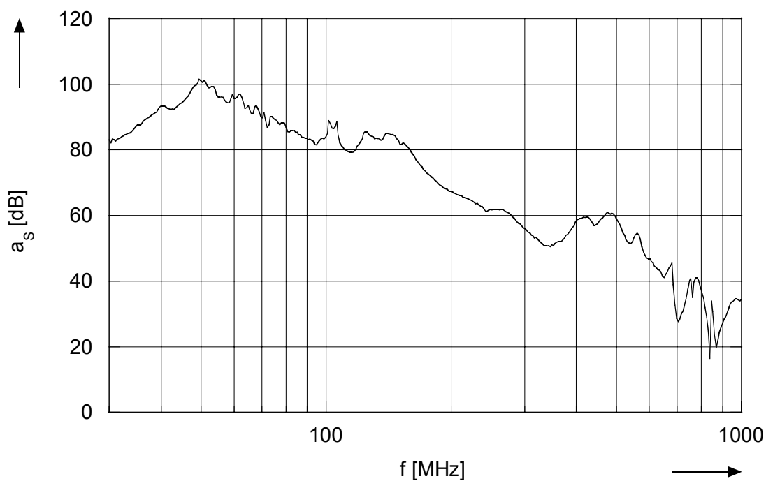
Bild 7: Schirmdämpfung im Bereich von 30 MHz bis 1 GHz, „Ratiopac pro geschirmt“, Einstrahlung auf die linke Seite, Polarisation vertikal.
