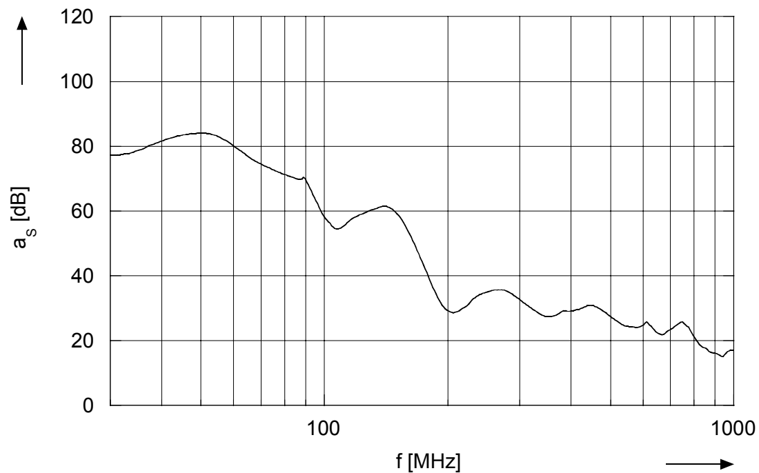
Bild 13: Typische Schirmdämpfung im Bereich von 30 MHz bis 1 GHz, „Ratiopac pro ungeschirmt“. Berechnet aus Worst Case der Kurven der Seitenwände, wobei Hohlraumresonanzen durch Glättung ausgeblendet wurden.
