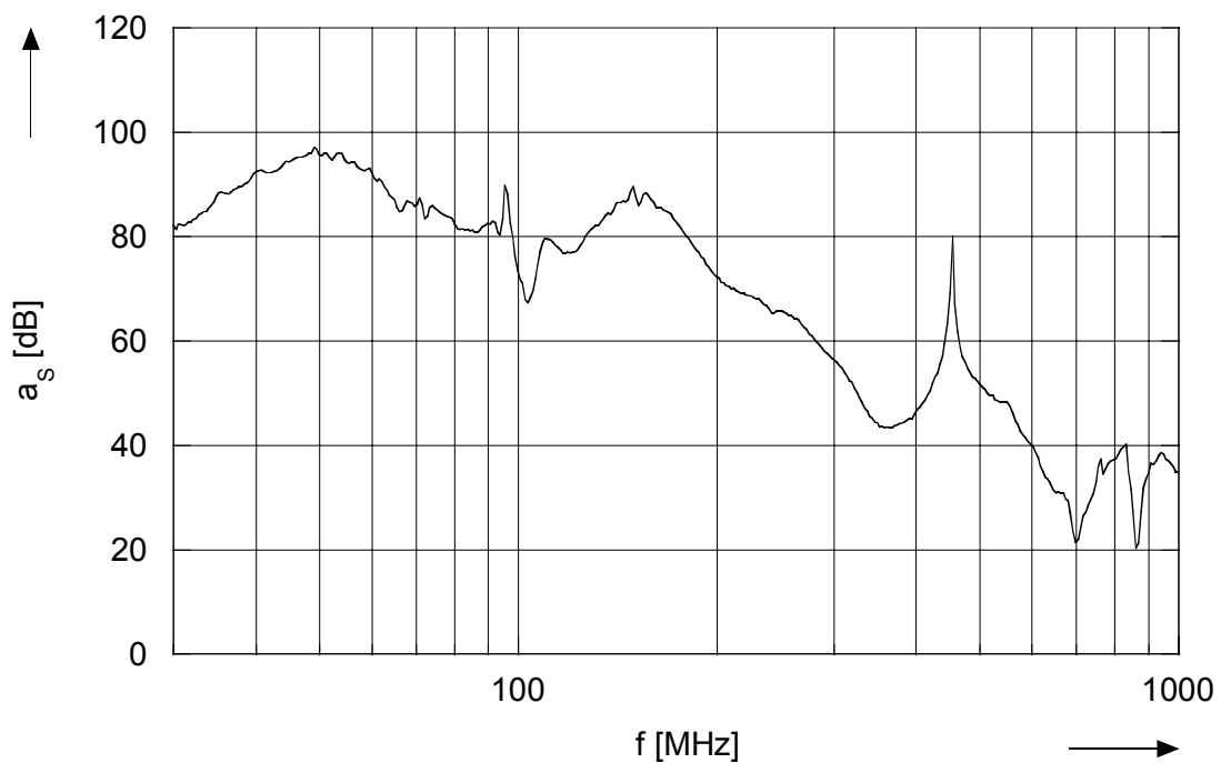
Bild 6: Schirmdämpfung im Bereich von 30 MHz bis 1 GHz, „Ratiopac pro geschirmt“, Einstrahlung auf die Rückseite, Polarisation vertikal.
