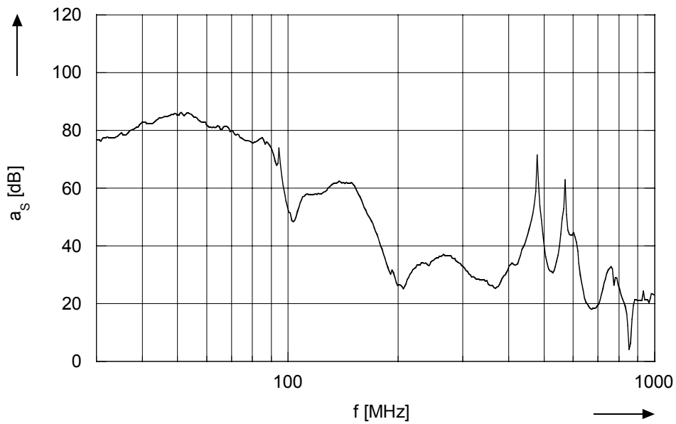
Bild 12: Schirmdämpfung im Bereich von 30 MHz bis 1 GHz, „Ratiopac pro ungeschirmt“, Einstrahlung auf die linke Seite, Polarisation vertikal.
