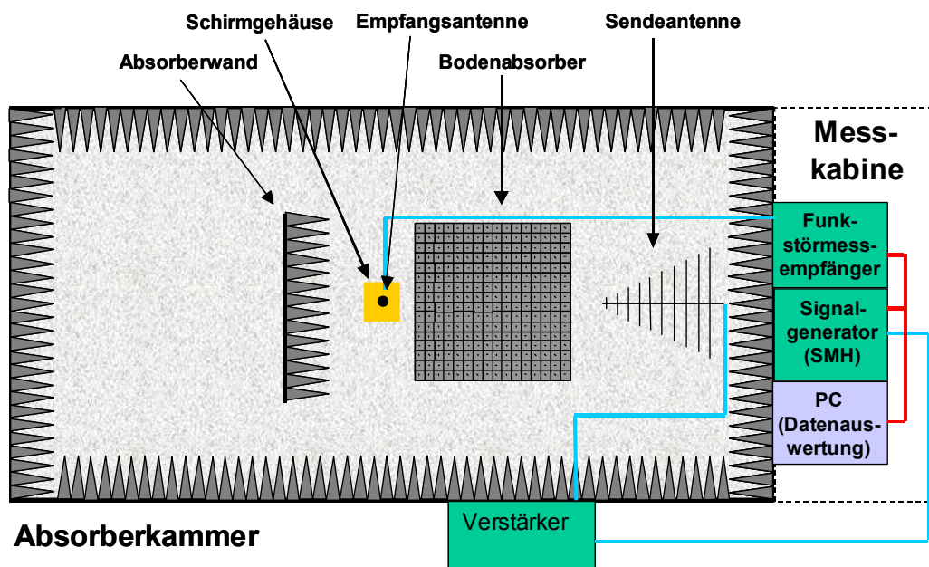
Bild 1: Schematischer Messaufbau der Schirmdämpfungsmessung.
