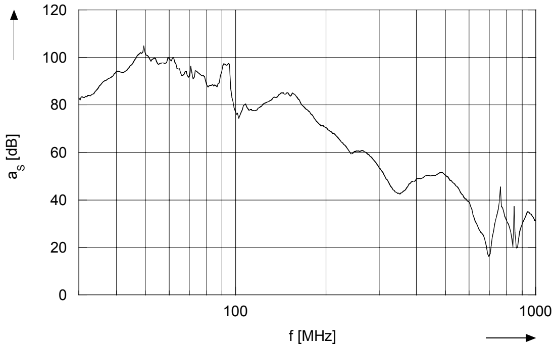
Bild 4: Schirmdämpfung im Bereich von 30 MHz bis 1 GHz, „Ratiopac pro geschirmt“, Einstrahlung auf die Frontseite, Polarisation vertikal.
