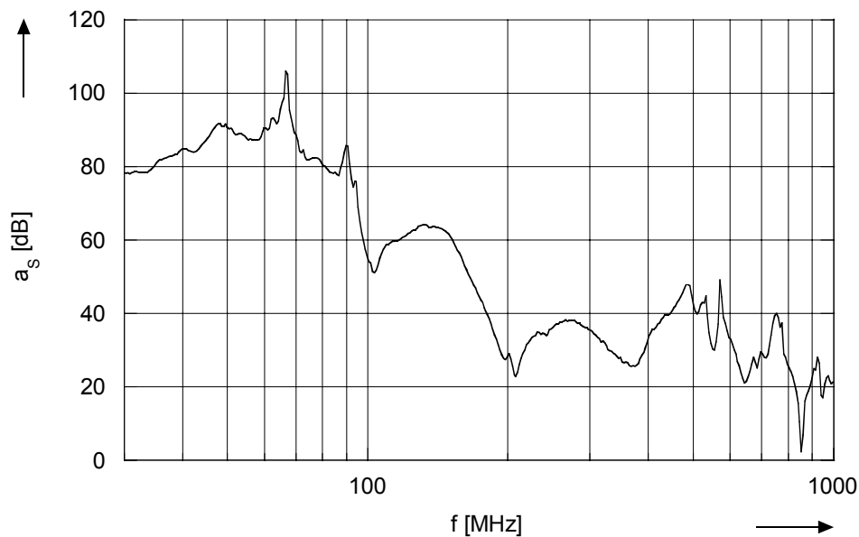
Bild 10: Schirmdämpfung im Bereich von 30 MHz bis 1 GHz, „Ratiopac pro ungeschirmt“, Einstrahlung auf die rechte Seite, Polarisation vertikal.
