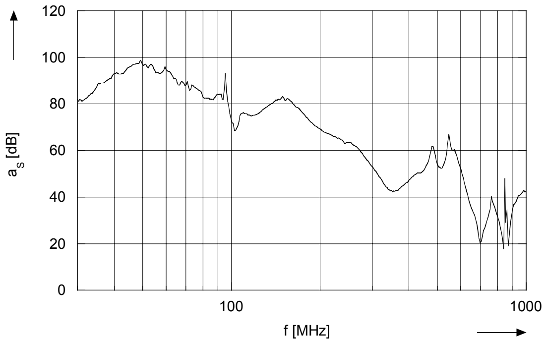
Bild 5: Schirmdämpfung im Bereich von 30 MHz bis 1 GHz, „Ratiopac pro geschirmt“, Einstrahlung auf die rechte Seite, Polarisation vertikal.
