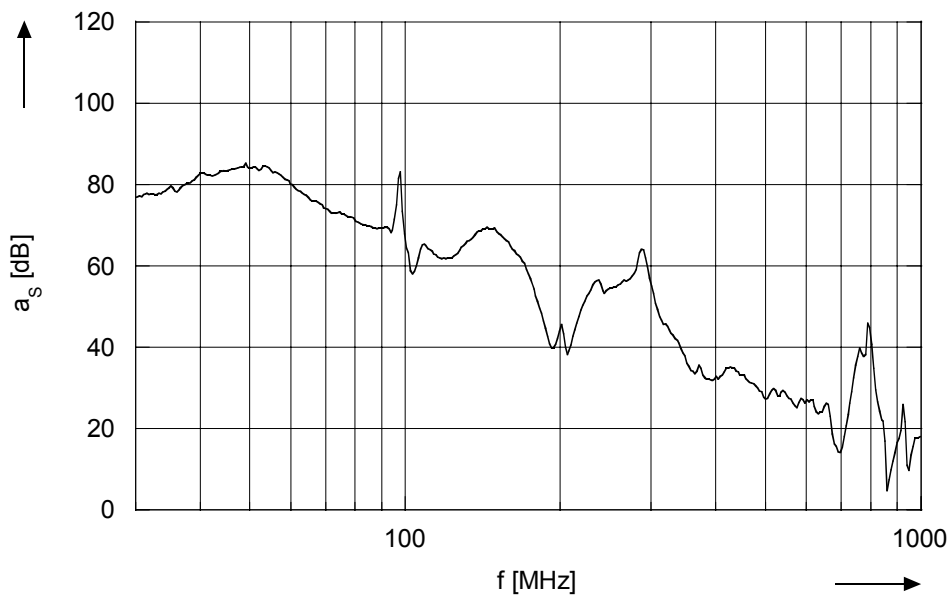
Bild 11: Schirmdämpfung im Bereich von 30 MHz bis 1 GHz, „Ratiopac pro ungeschirmt“, Einstrahlung auf die Rückseite, Polarisation vertikal.
