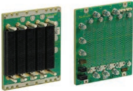
VPX Backplanes
