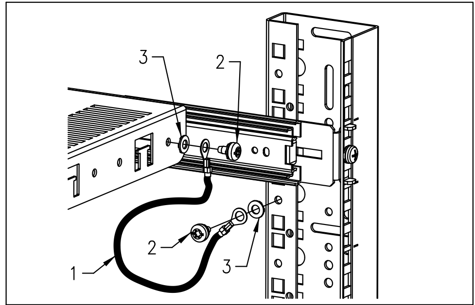
Montage auf Gestell On frame mounted Montage sur cadre
