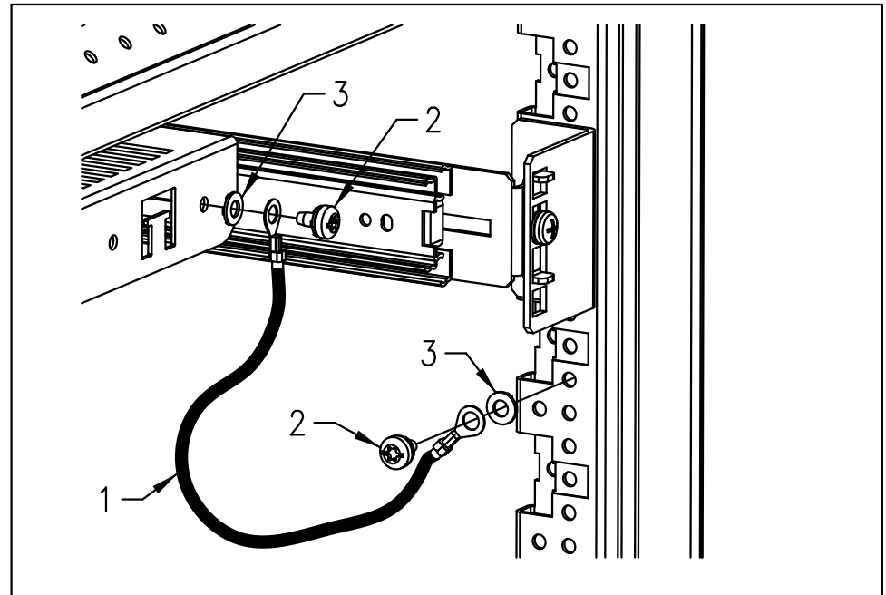
Montage auf Gestell On frame mounted Montage sur cadre
